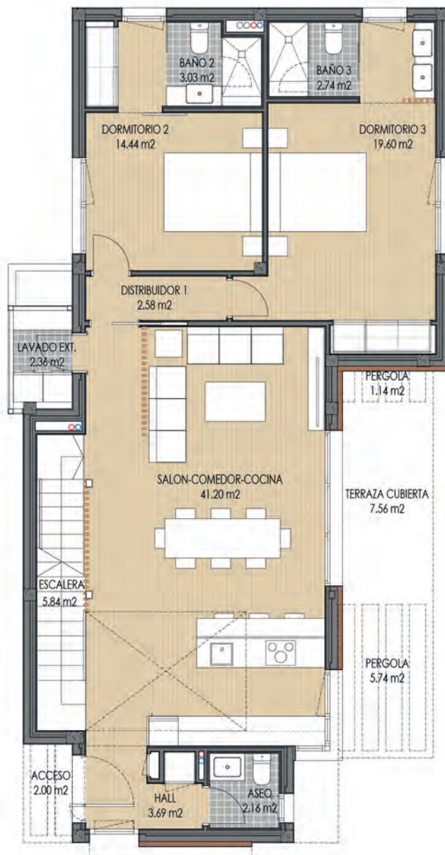
PLANTA BAJA
