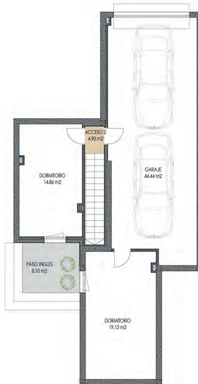
PLANTA SÓTANO
