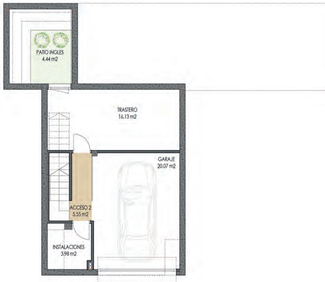
PLANTA SÓTANO
