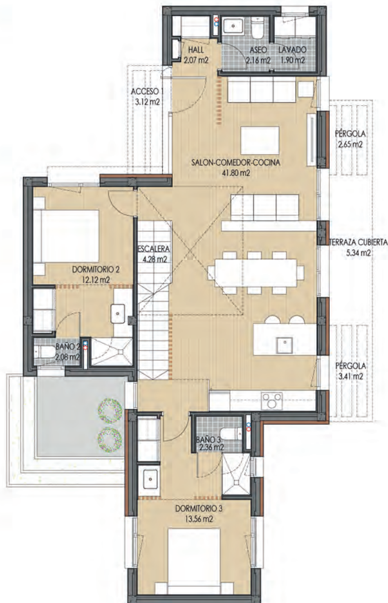
PLANTA BAJA
