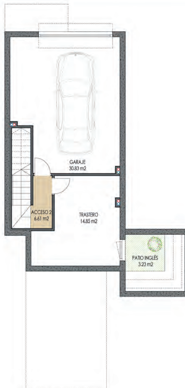
PLANTA SÓTANO
